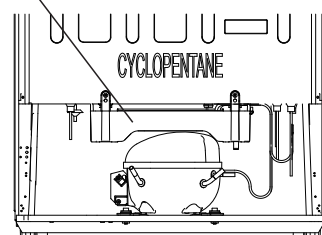
蒸発皿
