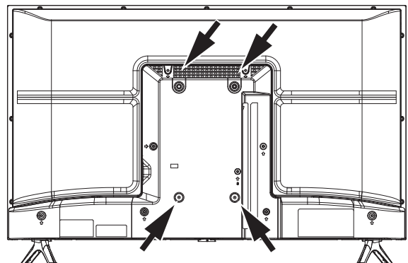
VESA規格 ねじ穴 (4カ所)
