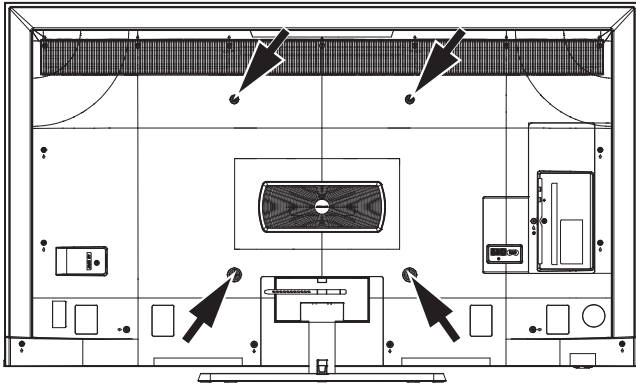
VESA規格 ねじ穴 (4カ所)
